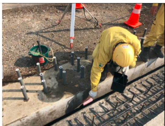
②ひび割れ部にローラーを使って、シリカを塗布
